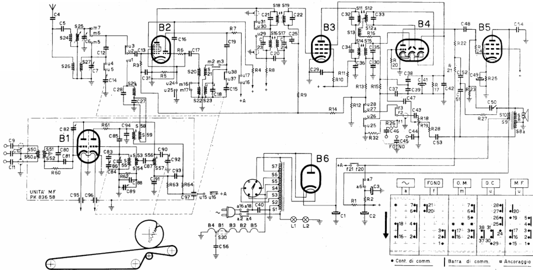
COMMUTATORE IN POSIZIONE D.C.
